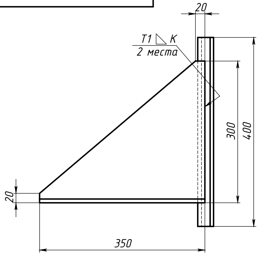
Поз.1 (Основание)
