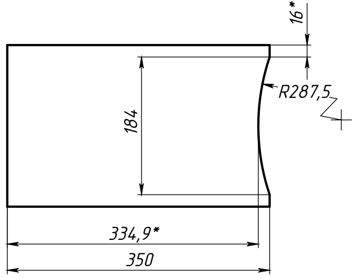
Поз.1 (Основание)
