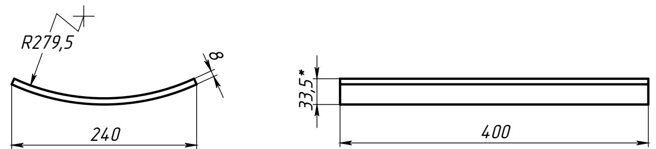
Поз.3 (Ложемент)
